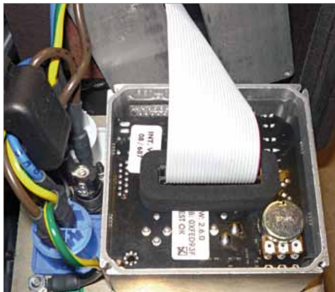
Procesor DSP zamknięto w szczelnej obudowie, z której sygnały wyprowadzono wiązką kablową.
